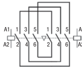
Diagrama elétrico
